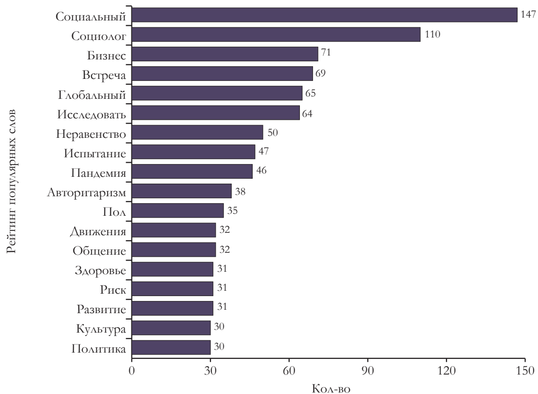
Рис. 2. Популярные слова Всемирного социологического конгресса 2023 г.
